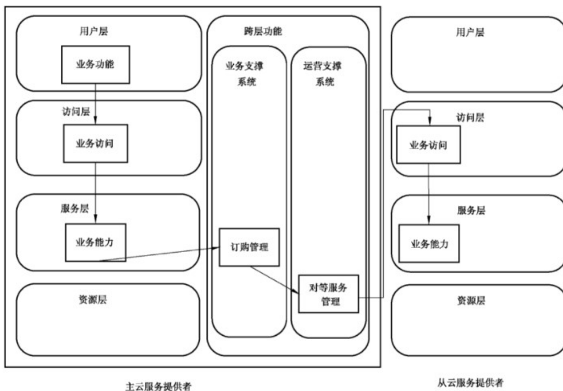
图 A.6 提供者和对等提供者之间的业务接口关系
