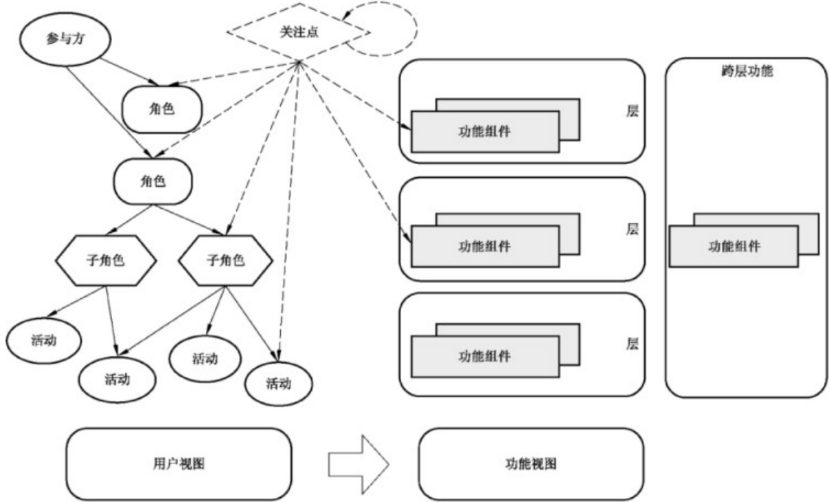
图 3 用户视图向功能视图的转换
