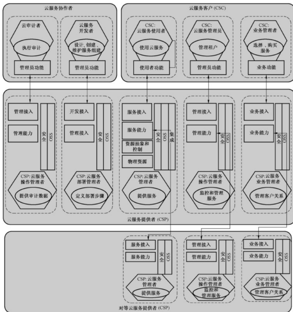
图 16 活动和组件之间关系和交换示例
